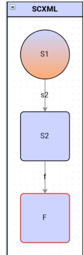
scxmlgui
