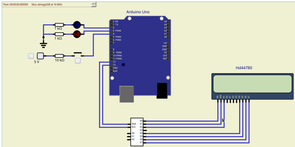
FIGURE 2 – Vue du câblage relative aux premières questions du TP1 dans SimulIDE
