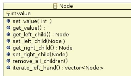
Figure 2: La classe Node
