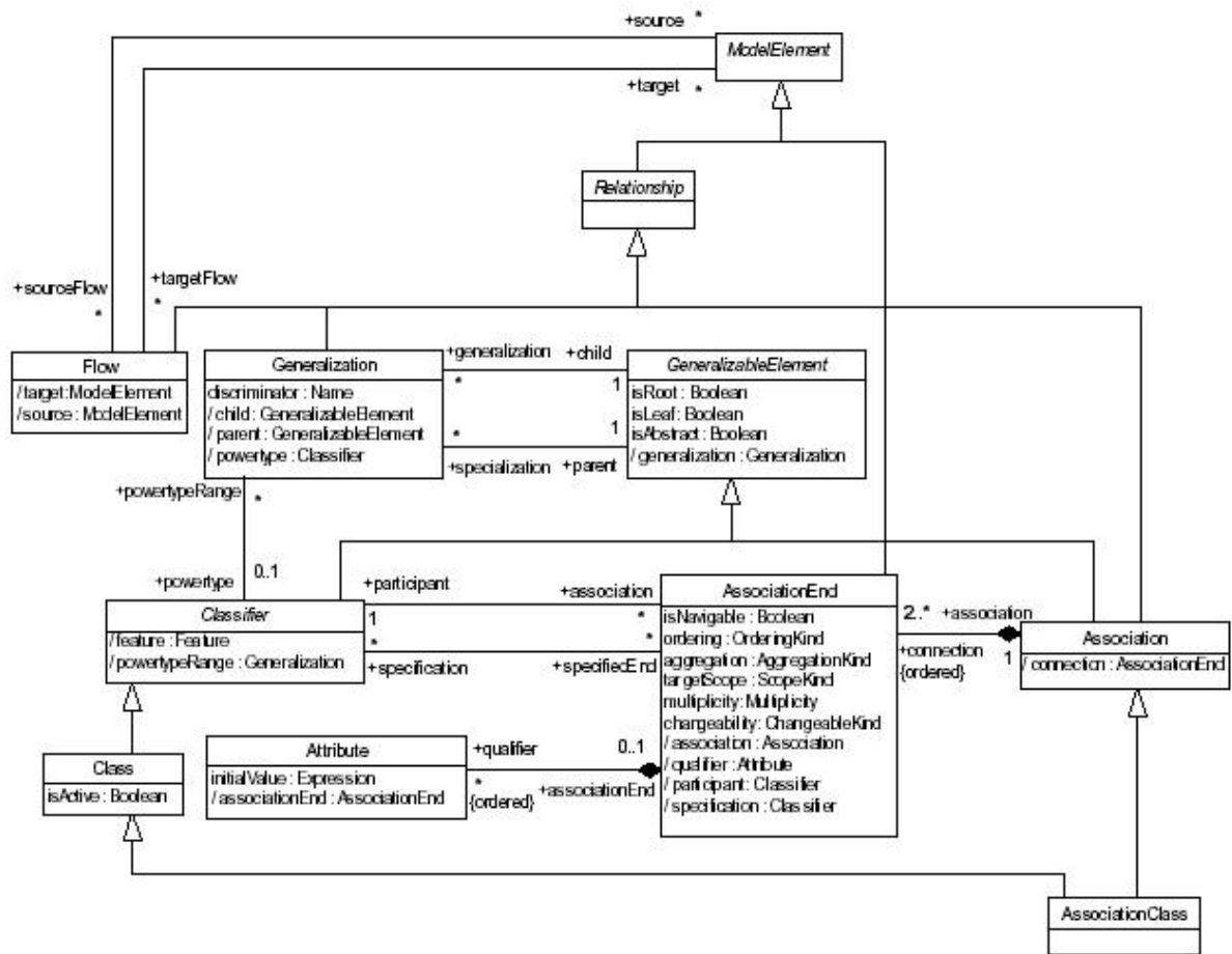
FIG. 5.6.: Le paquetage Core - Relationships d'UML
