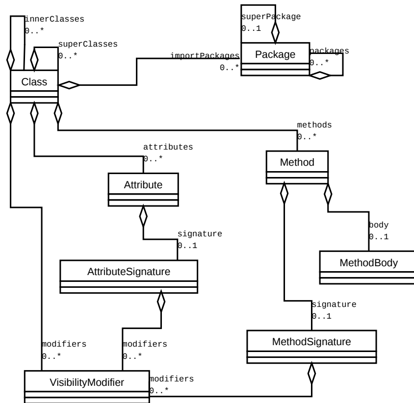
FIG. 3.1.: Concepts d'une préoccupation pris en compte pour la composition
