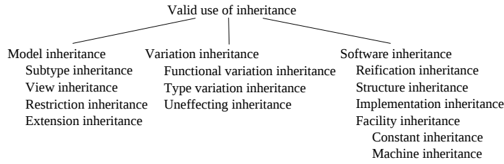
FIG. 5.11.: Taxinomie de l'héritage de Bertrand Meyer
