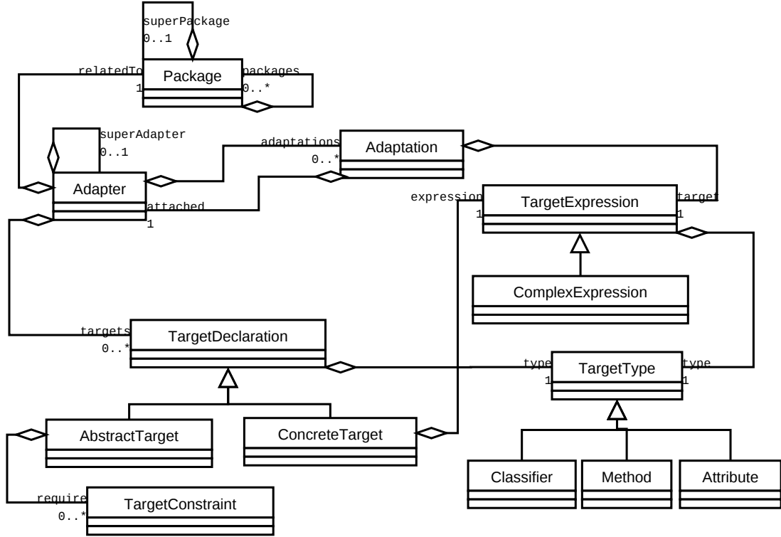
FIG. 3.2.: Réification de la composition de deux préoccupations
