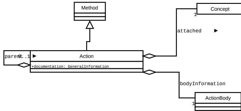
FIG. 6.11.: Description d'une action dans SmartModels
