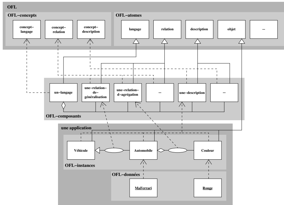
FIG. 4.2.: Architecture d'OFL
