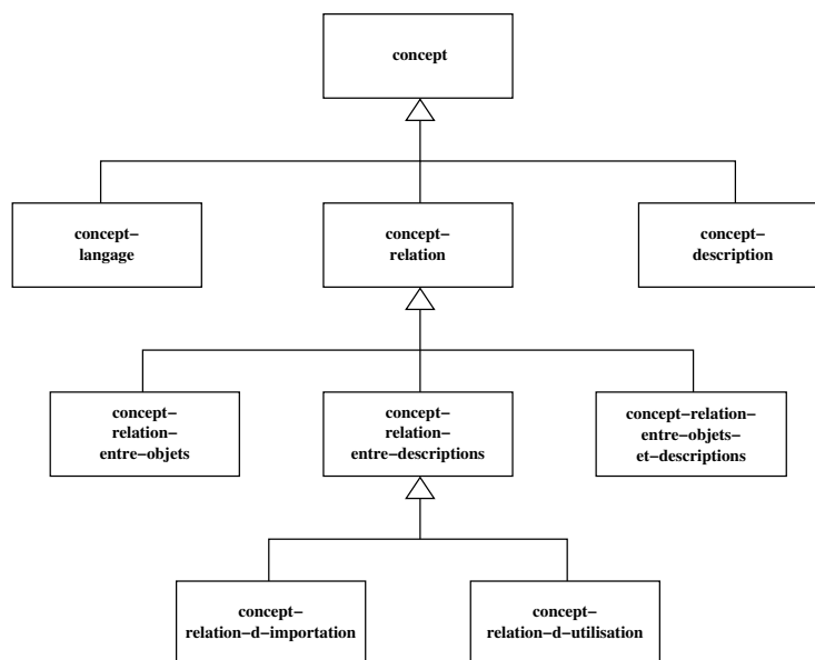
FIG. 4.3.: Les OFL-concepts
