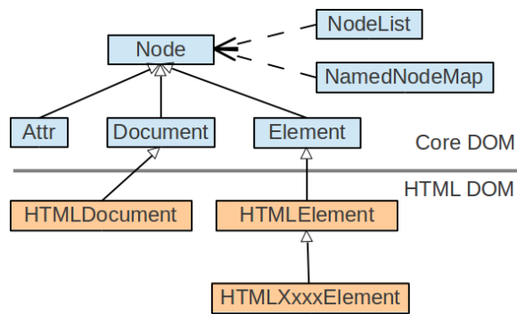
FIGURE 3.2 – Les objets DOM et leurs relations.
